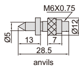
anvils
